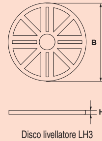
Disco livellatore LH3 Levelling disc LH3
